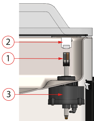
Schéma 2 : Aperçu du système de soudure (y compris le cylindre de soudure)
