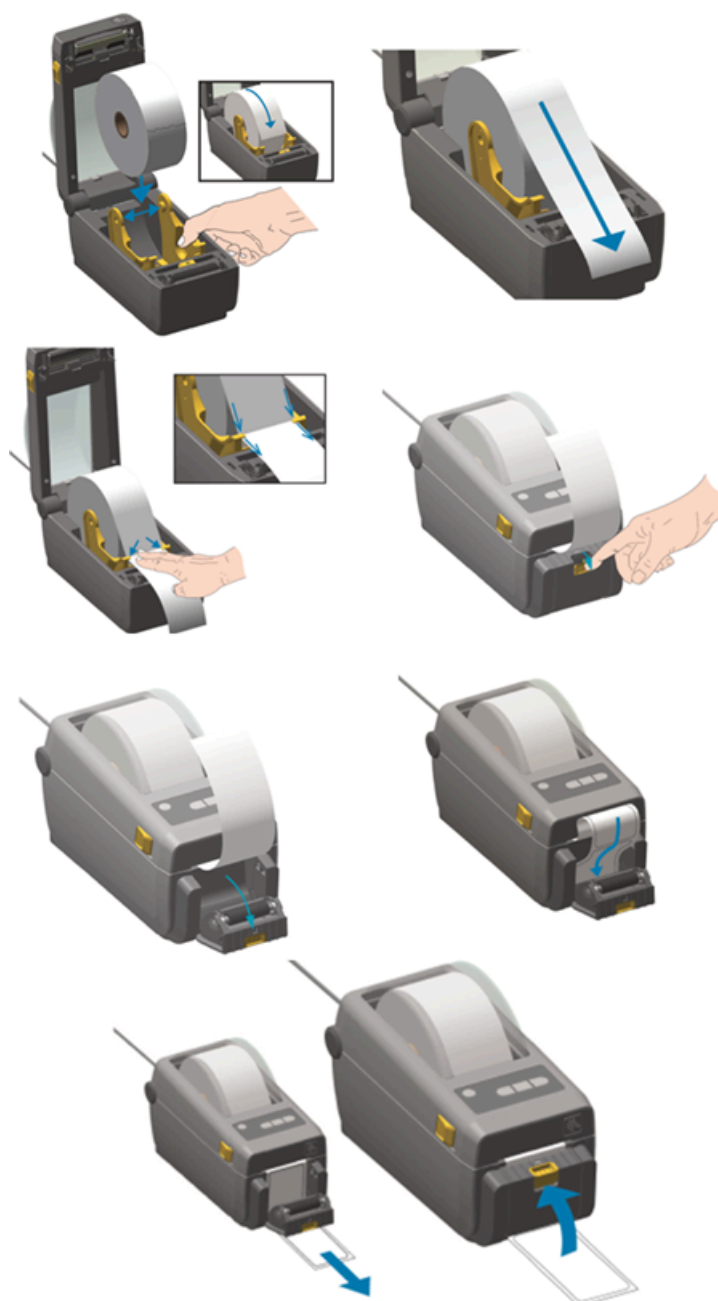
Schéma 13 : Remplacement du rouleau d'imprimante
