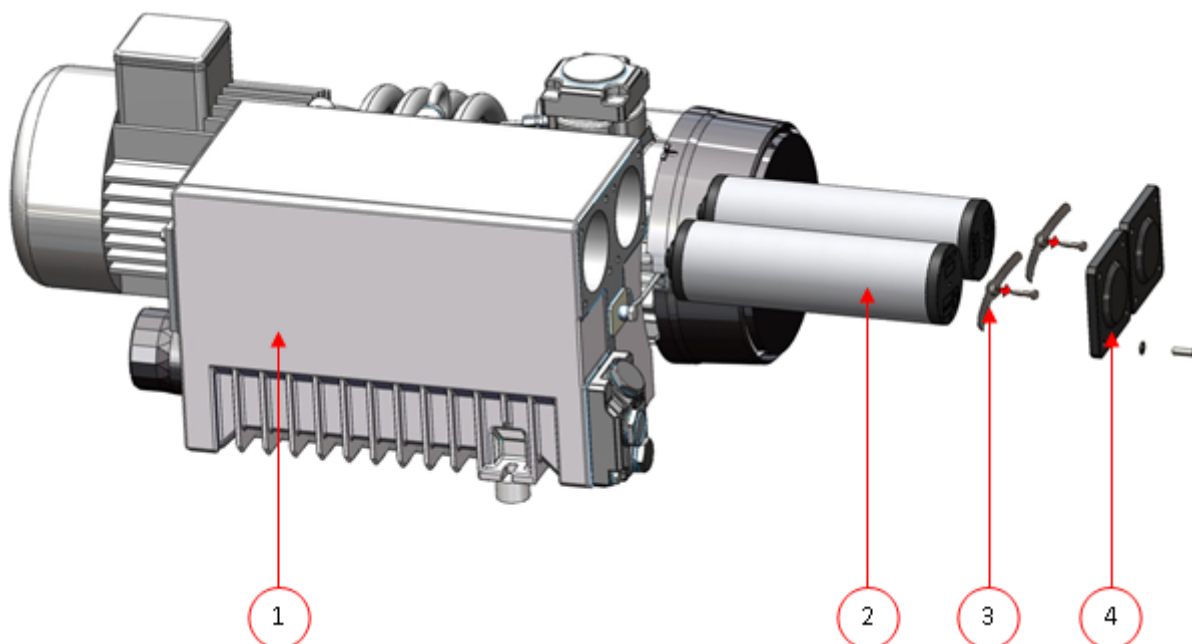
Schéma 23 : Remplacement du filtre à échappement d'air
