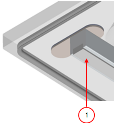
Schéma 18 : Remplacement du silicone des contre-barres
