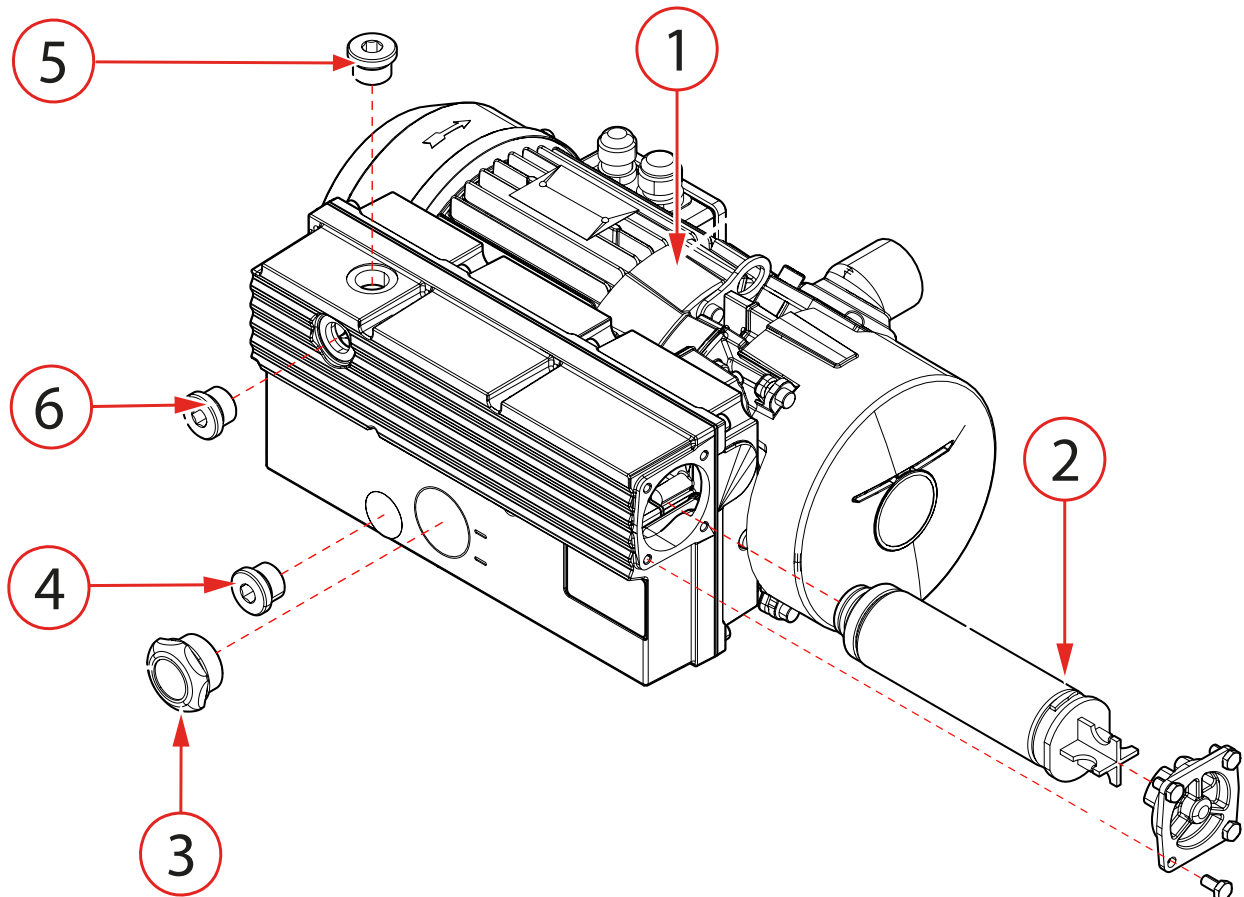
Schéma 20 : Aperçu de la pompe Becker
