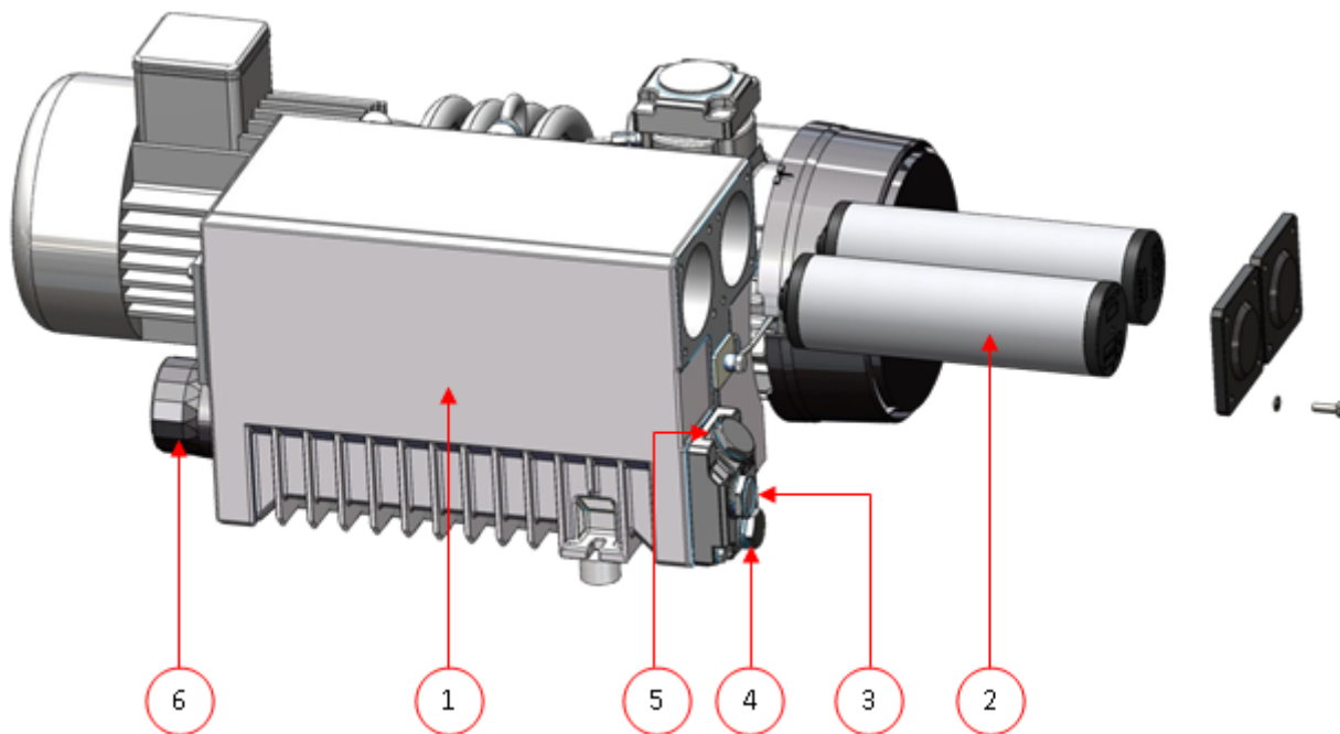
Schéma 22 : Aperçu de la pompe Busch
