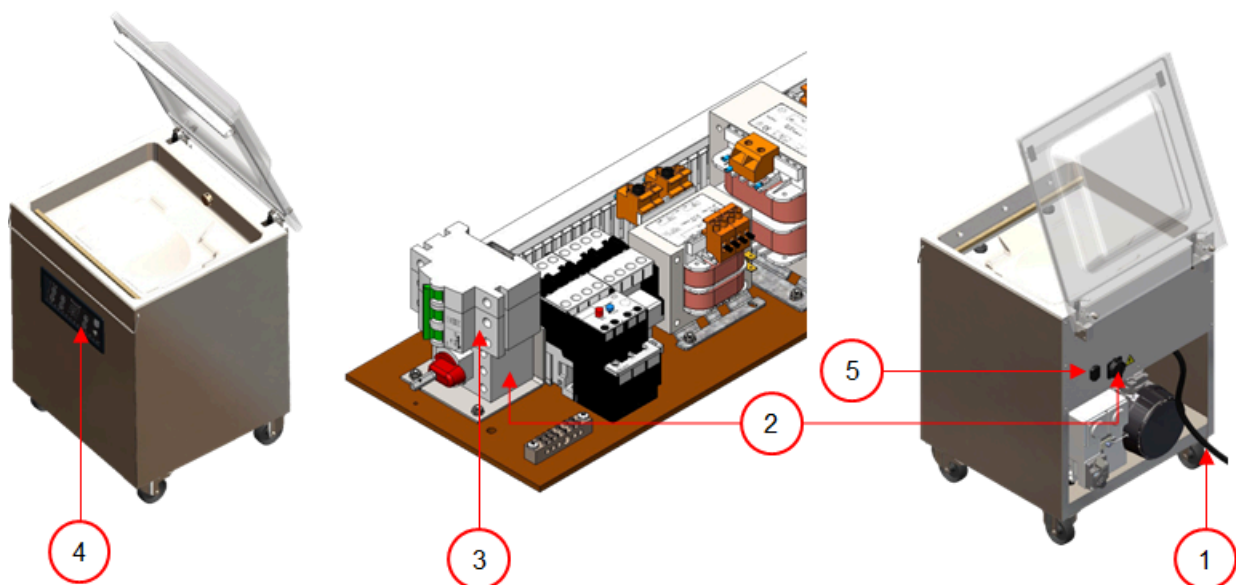
Schéma 24 : Aperçu de l'installation électrique, Marlin
