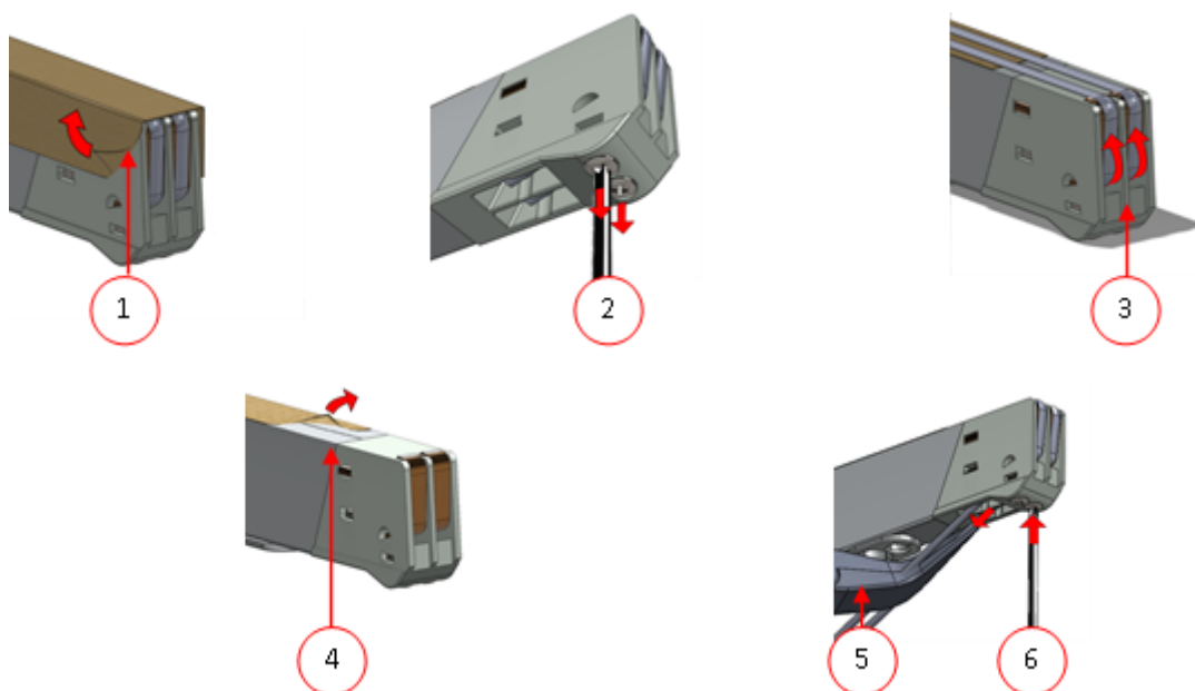
Schéma 17 : Remplacement de la résistance de soudure
