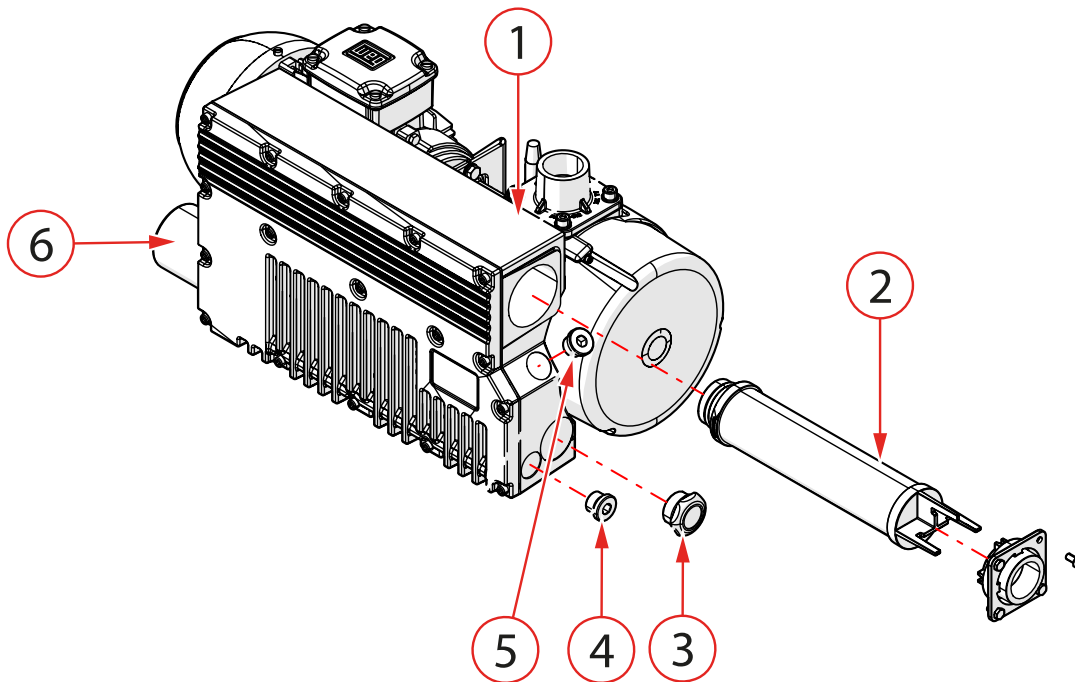
Schéma 21 : Aperçu de la pompe Becker
